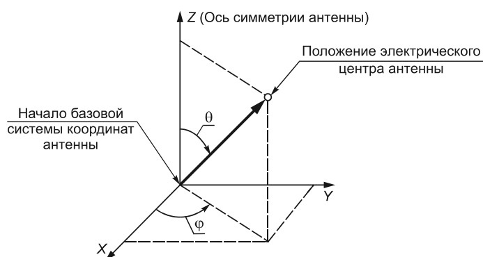
Рисунок 1 — Базовая система координат
